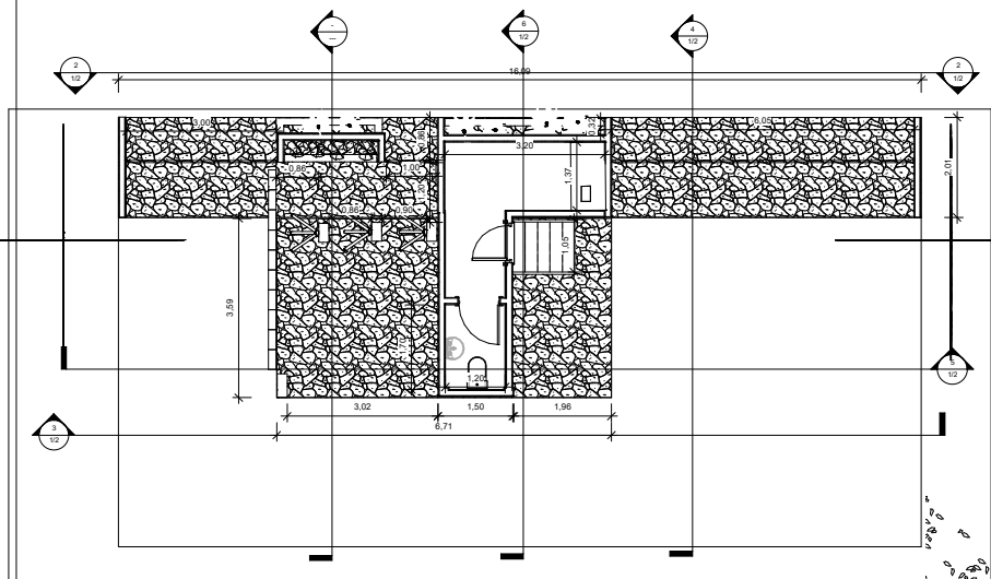
1 01 - térreo 1 : 50
