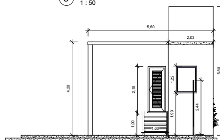
4 corte B 1 : 50
