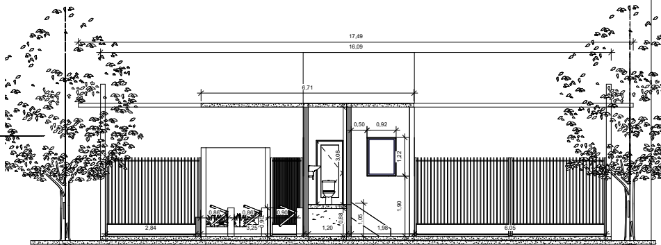
5 corte A 1 : 50
