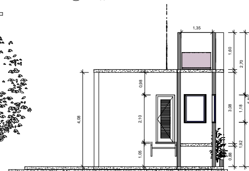
6 corte C 1 : 50
