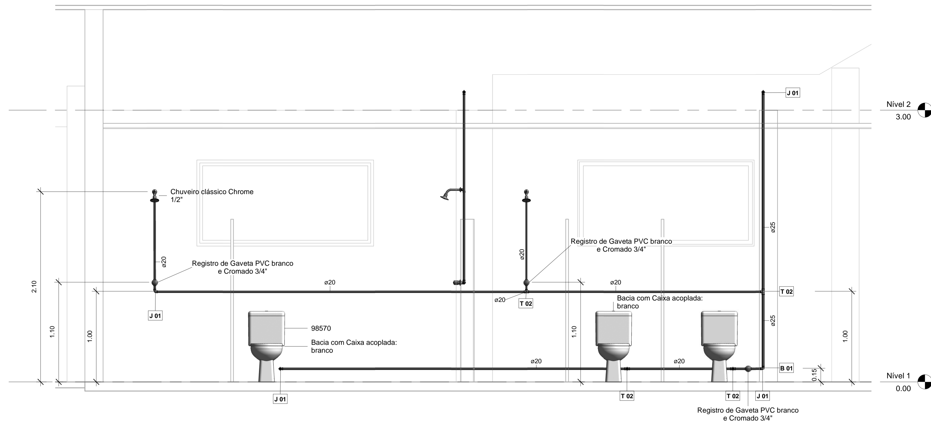
BB CORTE BB 1 : 20
