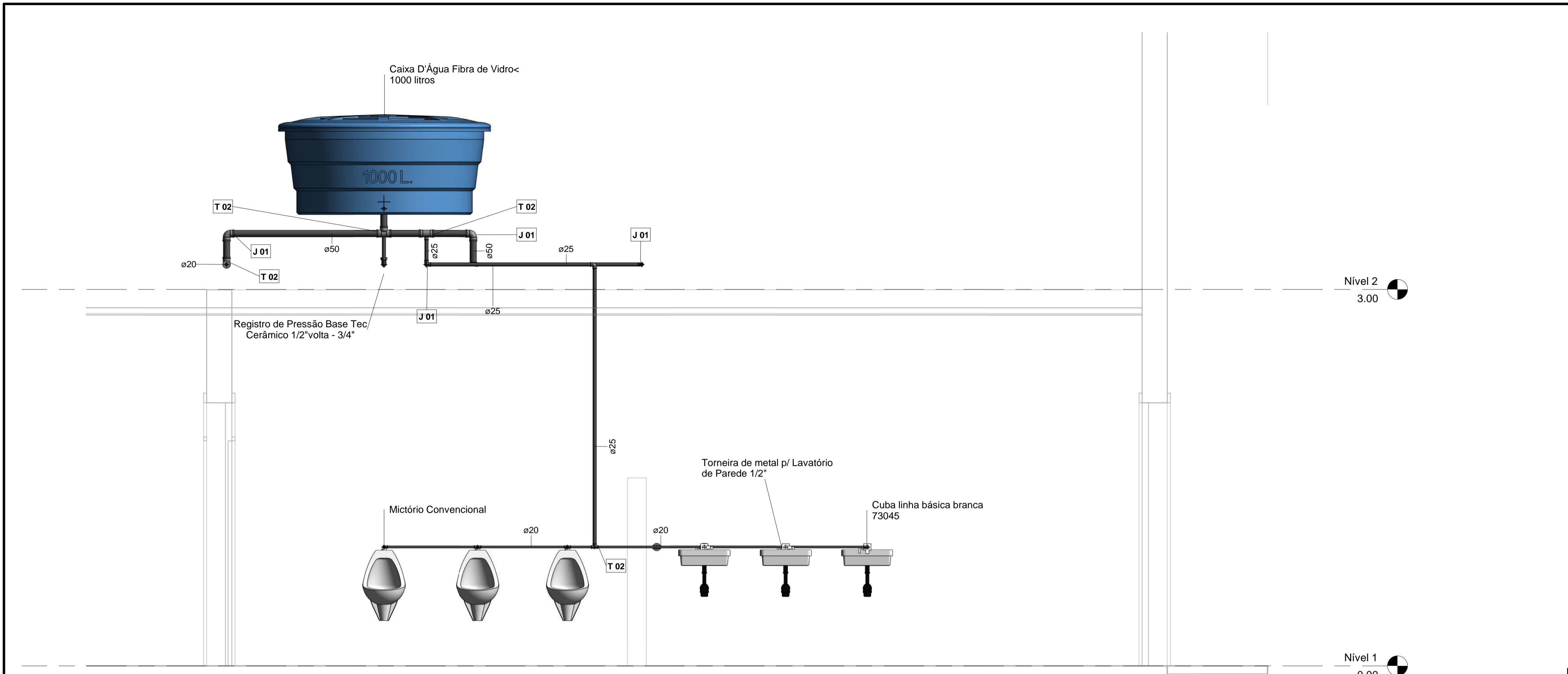
DD CORTE DD 1 : 20
